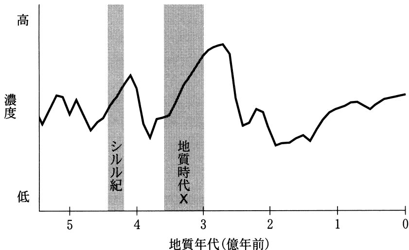
図 1 顕生代における地球大気中の ア 濃度の時間変化
